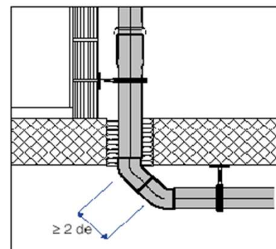
Esempio curva di collegamento colonna di scarico collettore sub orizzontale
