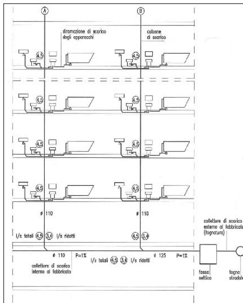
Schema impianto di scarico e collegamento alla fognatura
